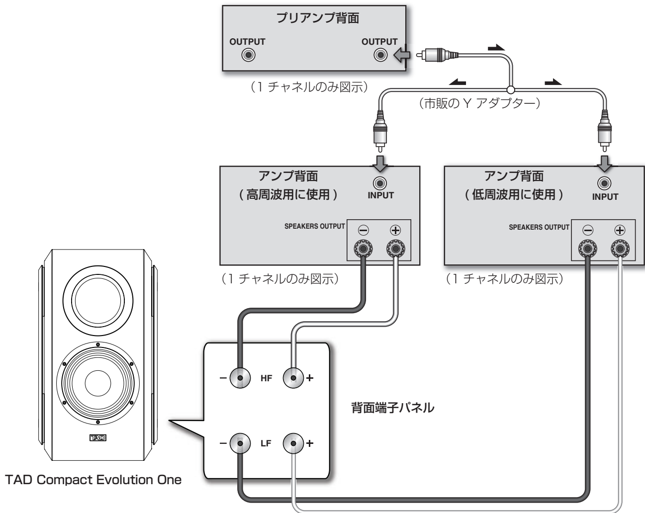
第 5 図 : TAD Compact Evolution One の 水平バイアンプシステム接続
