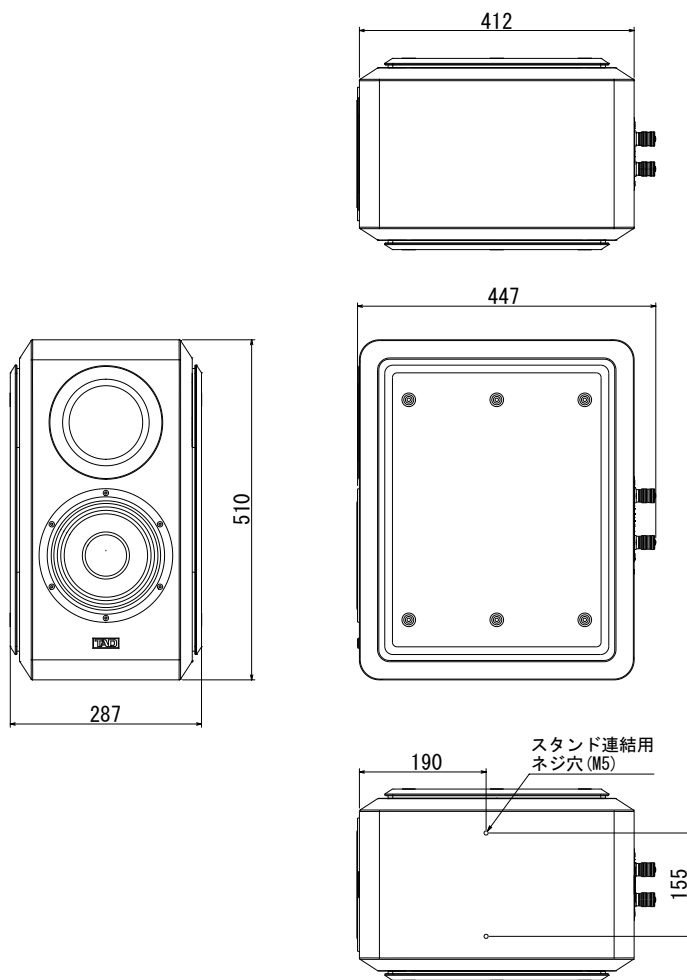
第6図：TAD Compact Evolution One スピーカーシステムの外形寸法
