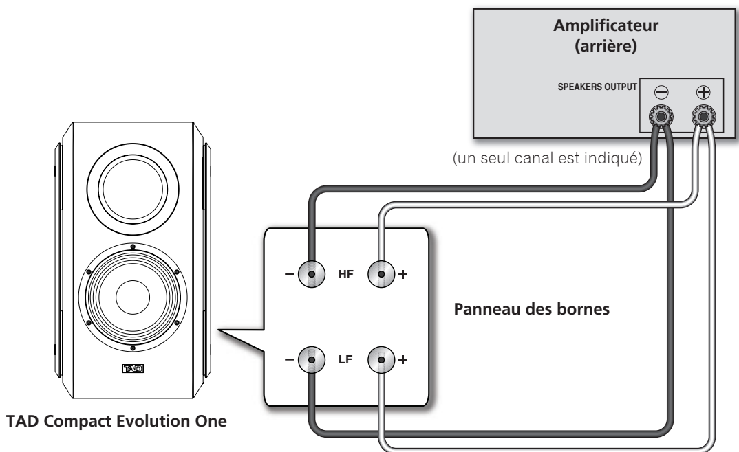
Figure 3. Connexion d'une enceinte TAD Compact Evolution One en un circuit bi-filaire
