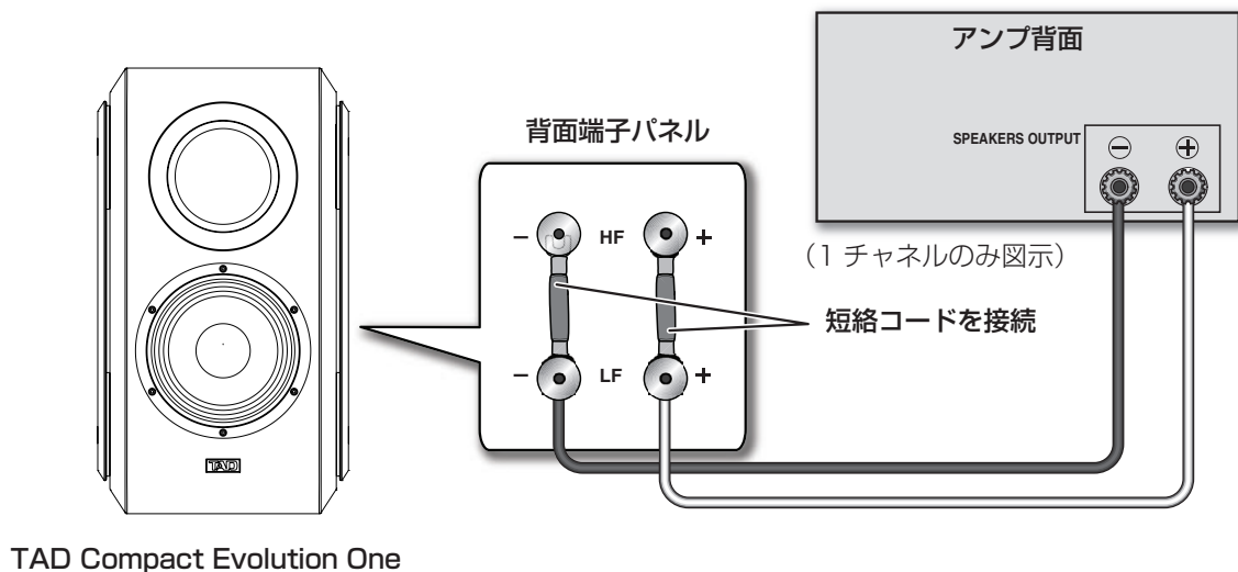
第 2 図 : TAD Compact Evolution One の シングルワイヤリング接続
