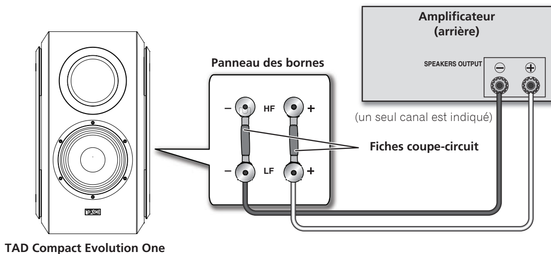
Figure 2. Connexion d'une enceinte TAD Compact Evolution One en un circuit unifilaire
