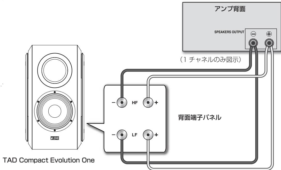
第 3 図：TAD Compact Evolution One のバイワイヤリング接続
