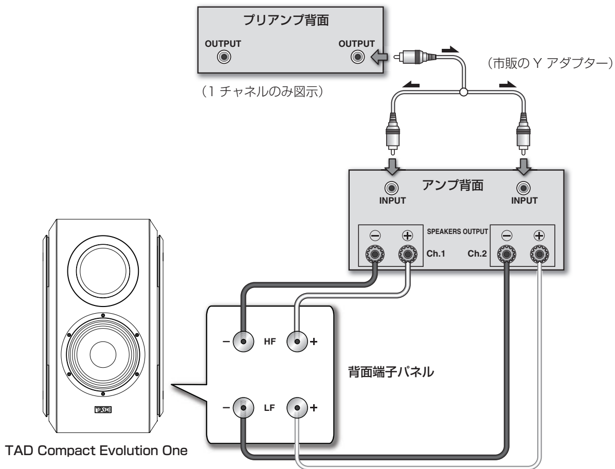
第 4 図：TAD Compact Evolution One の バーチカルバイアンプシステム接続
