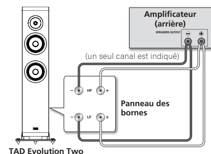
Figure 3. Connexion d'une enceinte en un circuit bi-filaire
