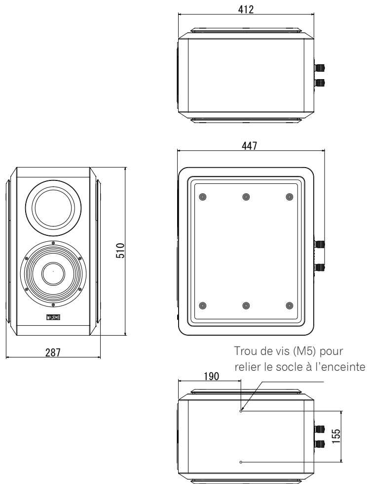
Figure 6 : Dimensions hors-tout de l'enceinte TAD Compact Evolution One
